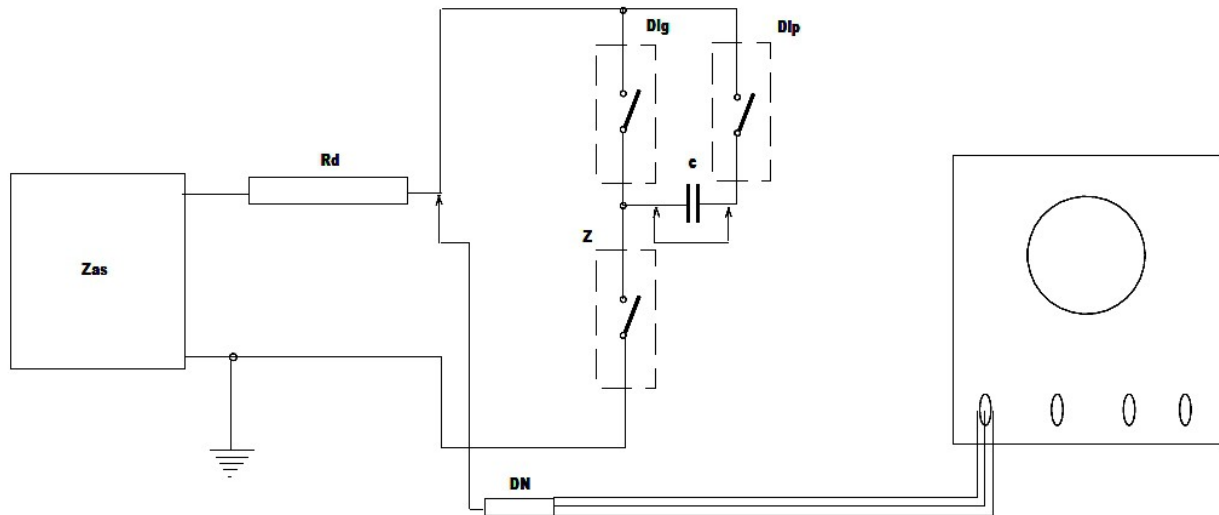
Schemat układu do próby czasów wyłącznika.
