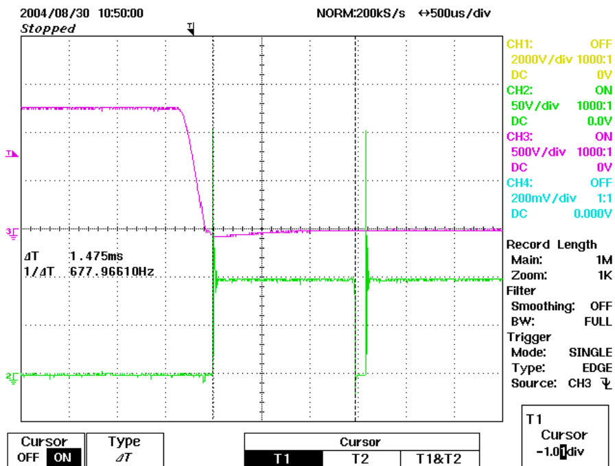
Oscylogram wynikowy do pomiaru czasów własnych.
